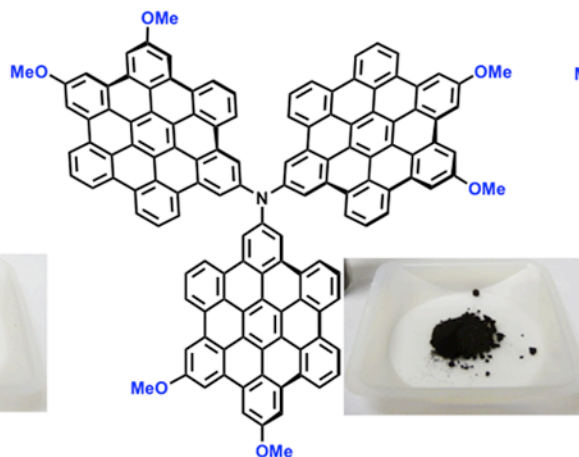
HBC-OMe
