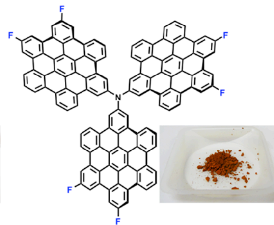
HBC-F
