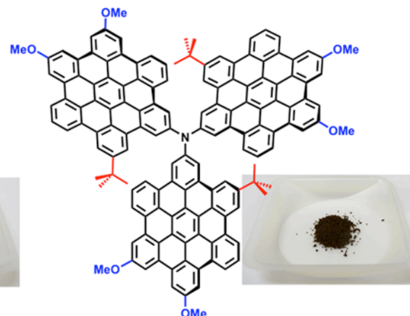
HBC-tBuOMe
