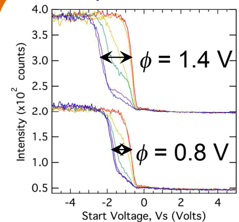
CuInGaSe 2 p-n profiles
