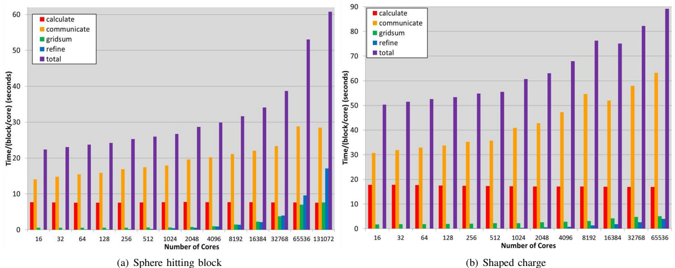
Fig. 5. miniAMR scaling
