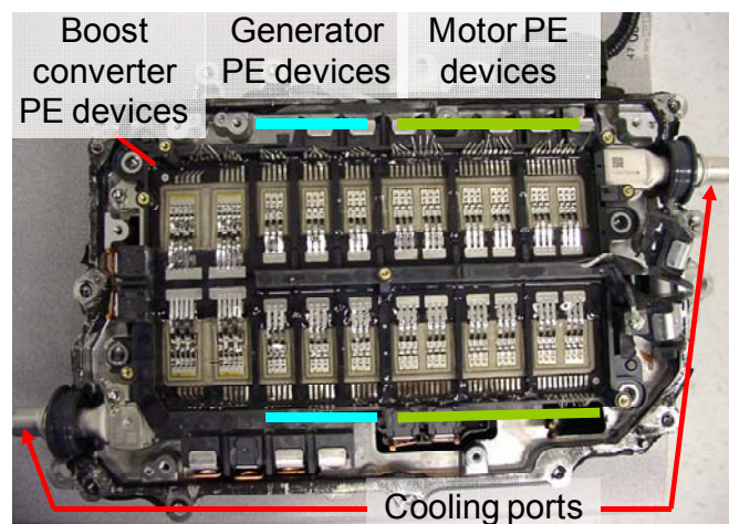
Fig. 3. 2010 Prius PEM.
