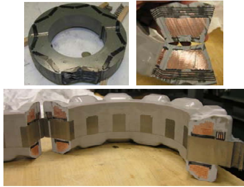
Fig. 10. 2010 Prius generator.
