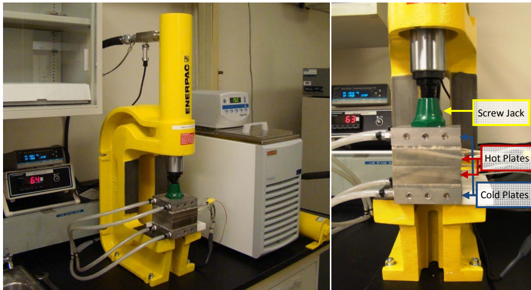
Fig. 54. NREL hot press
