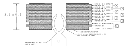
Press Fit Pin Interface
