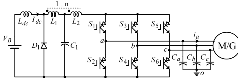
Fig. 5. CF-trans-ZSI.
