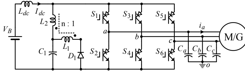
Fig. 4. CF-trans-qZSI.
