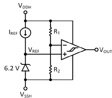
Fig. 16. UVLO topology.
