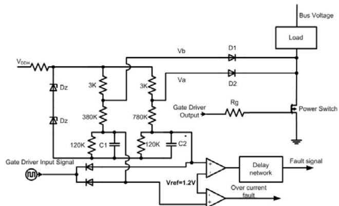
Fig. 26. Desaturation SCP.
