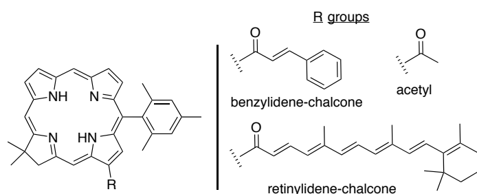
Chart 5. Chlorin-chalcones.
