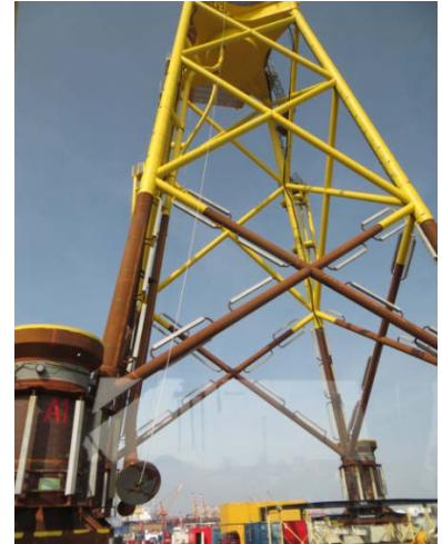
Fig. 2.5.1 Weserwind Jacket – Port of Bremerhaven GmbH
