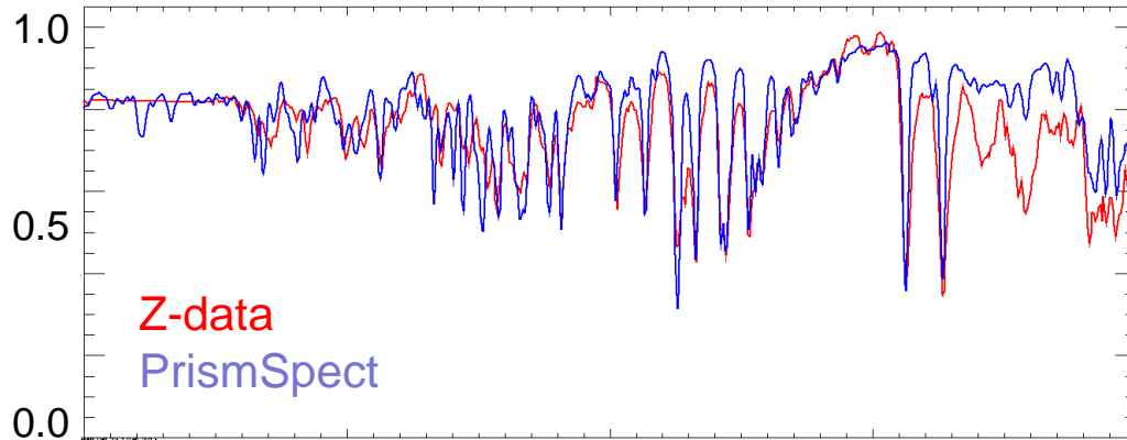
Thin Tamper* ( 156 \text{ eV} , 6.9 \times 10^{21} \text{ cm}^{-3} )
