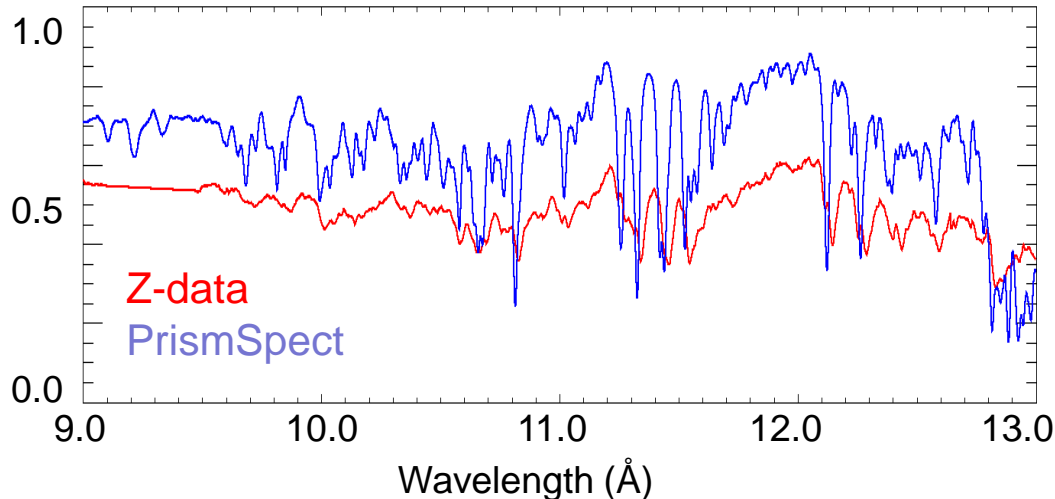
Thick Tamper ( 182 \text{ eV} , 31 \times 10^{21} \text{ cm}^{-3} )
