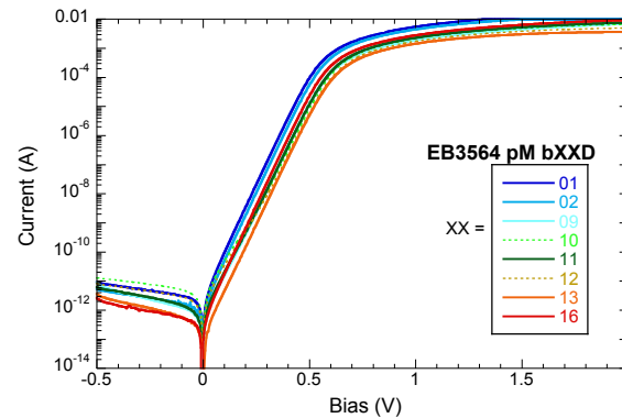
Diode I-V
