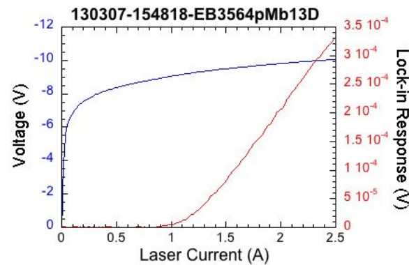
Pulsed Laser L-I-V
