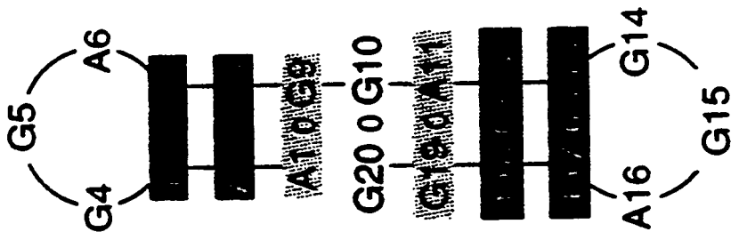
(AATGG) 4 A Stem-Loop Motif
