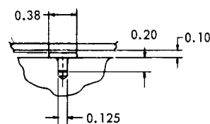
DETAIL-C TYP 120 PL
