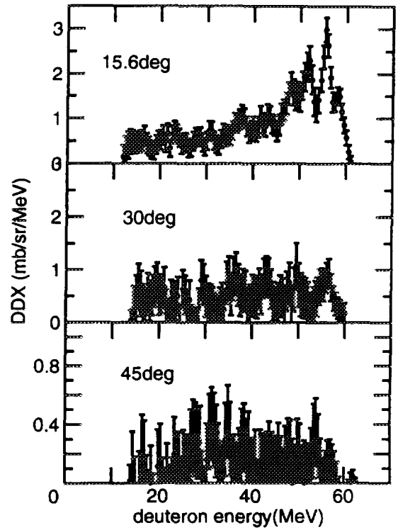
Fig. 7b Al(n,xd) DDX
