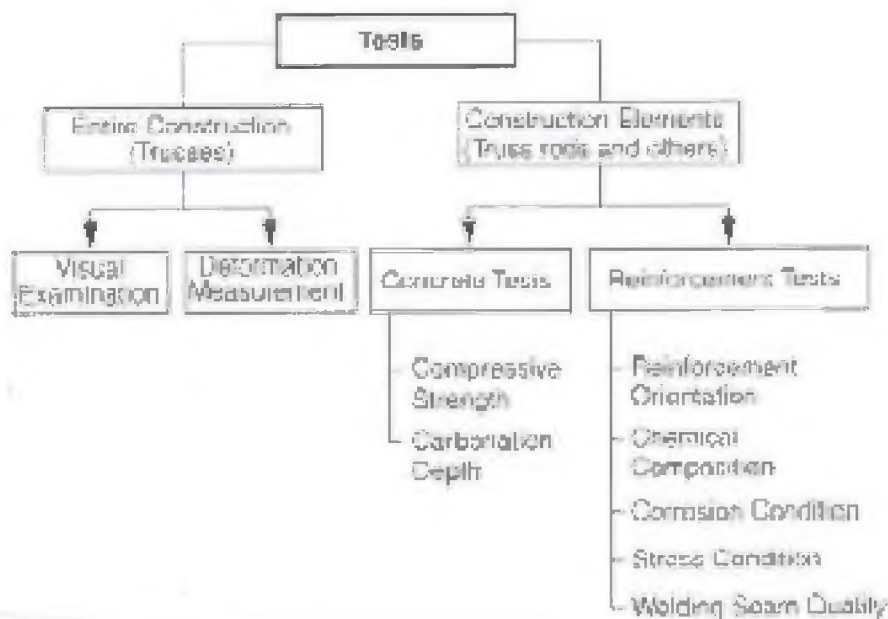
FIG. 17.6. Test programme.
